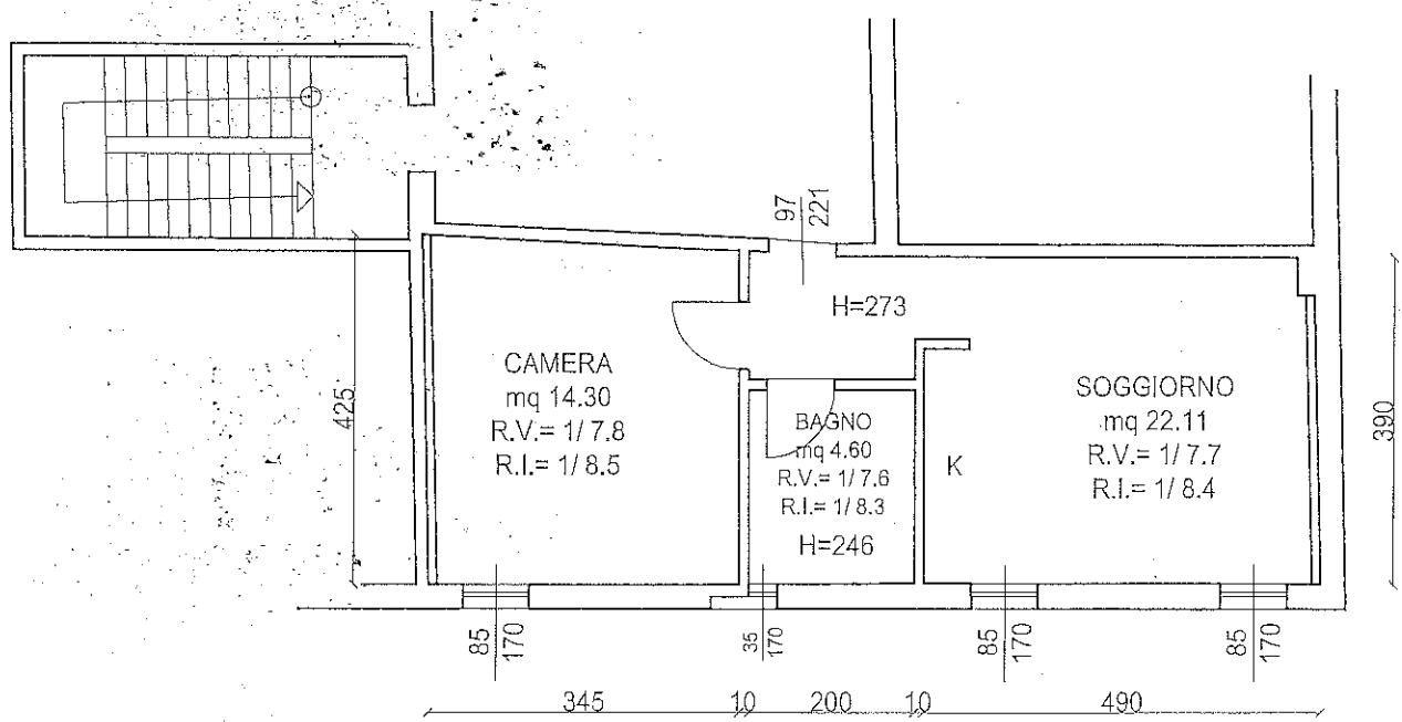
pianta piano secondo scala 1:100
